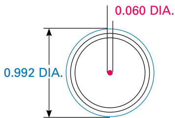
1/8" MINI TC
