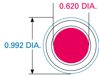
3/4" MINI TC
