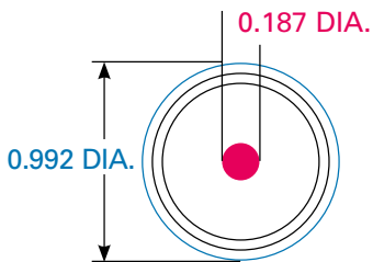
1/4" MINI TC
