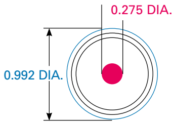
3/8" MINI TC
