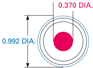
1/2" MINI TC
